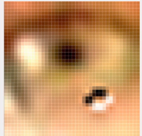
Bicubic
